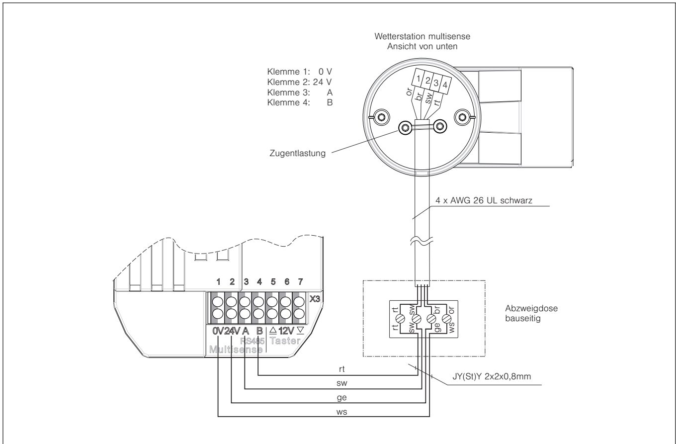
Abb. 14 Anschluss einer Wetterstation multisense
