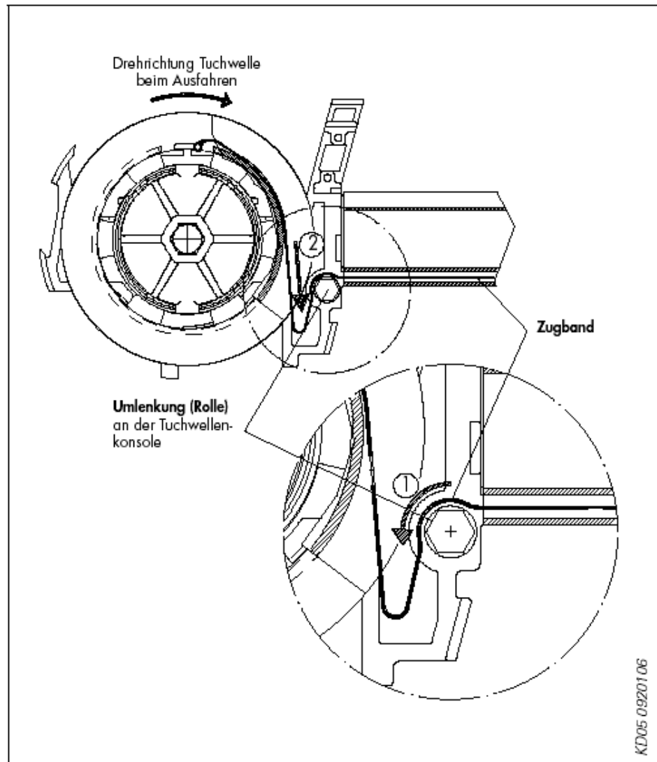
Bild 6: Zugbandumlenkung
