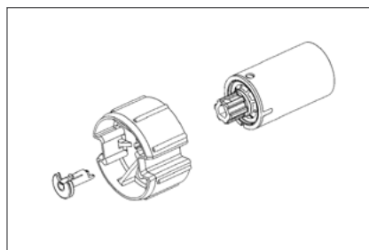
Afbbeelding 2: Koppelingsbeveiliging*
