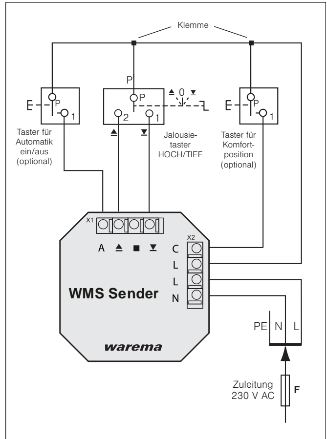
Abb. 3 Anschluss bei Steuerung von Sonnenschutzantrieben
