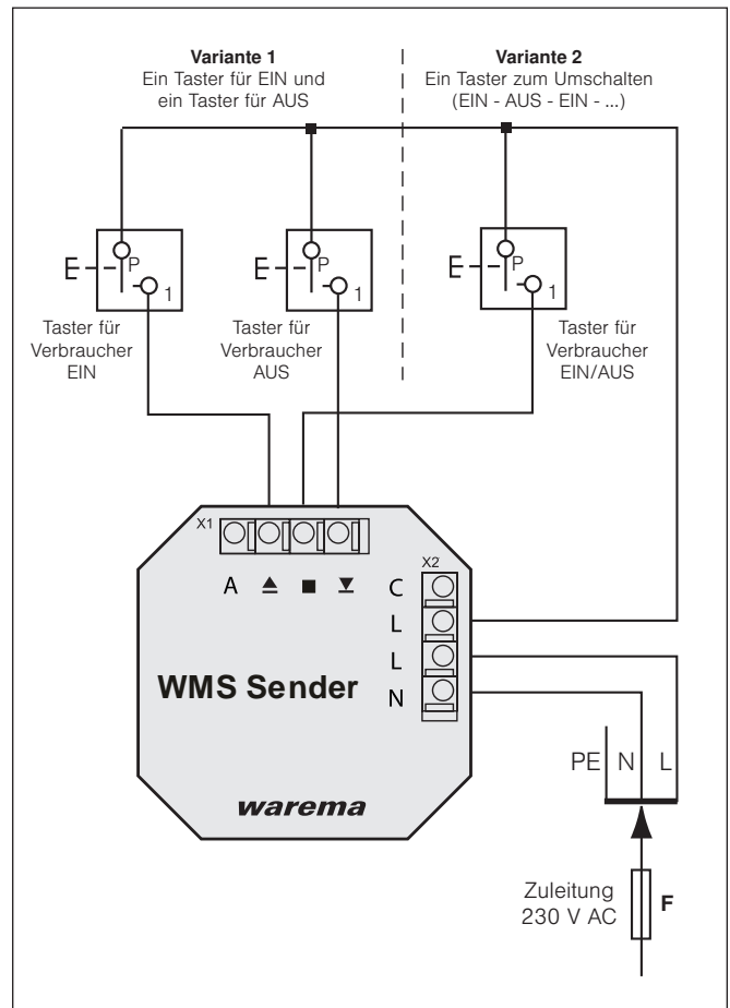
Abb. 4 Anschluss bei Steuerung von anderen Verbrauchern (z. B. Licht)
